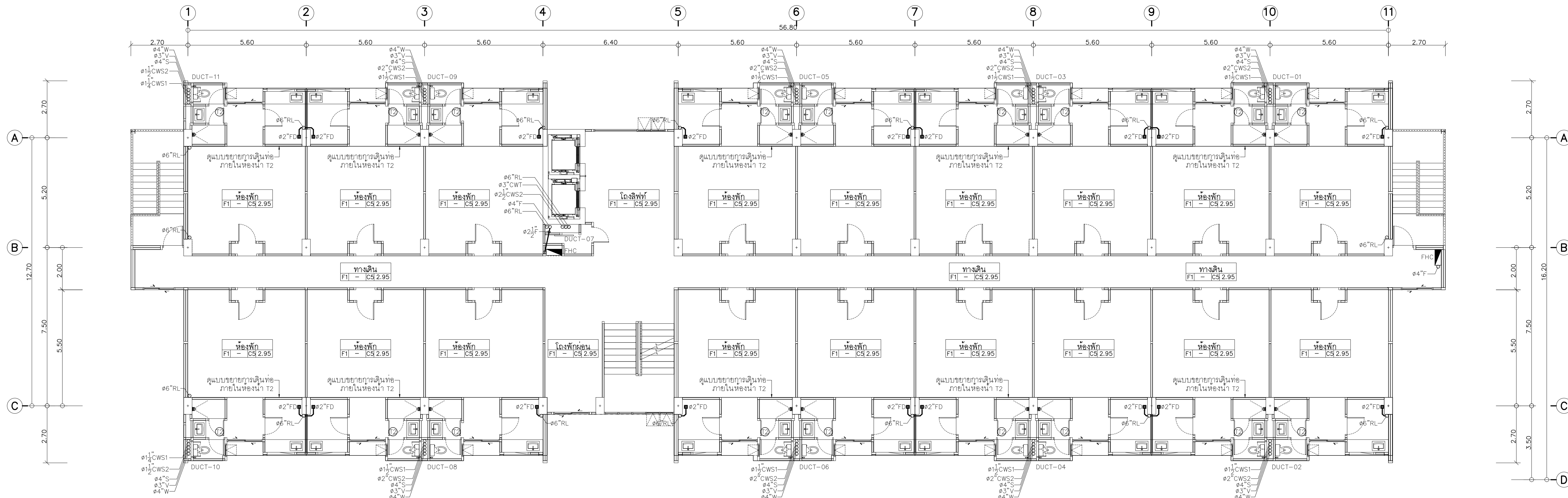
แปลนระบบสุขาภิบาลพื้นที่ 6
